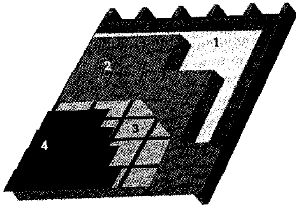
1. Dampscherf | 2. Isolatie | 3. Onderdak | 4. Dakbedekking
